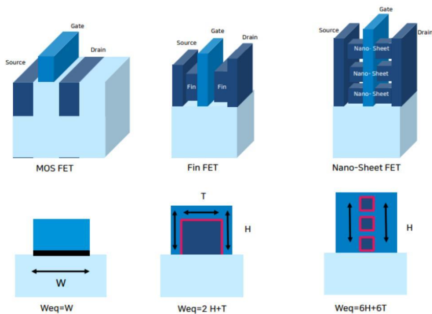
그림 15. Planar FET, MOSFET, GAAFET 구조 비교
