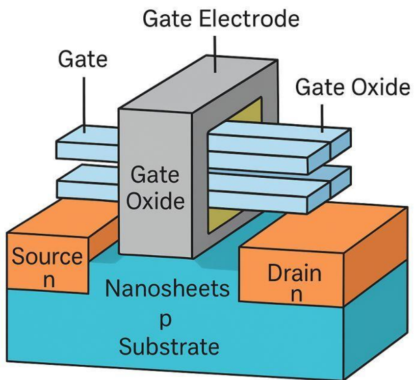
Gate-all-Around FET
